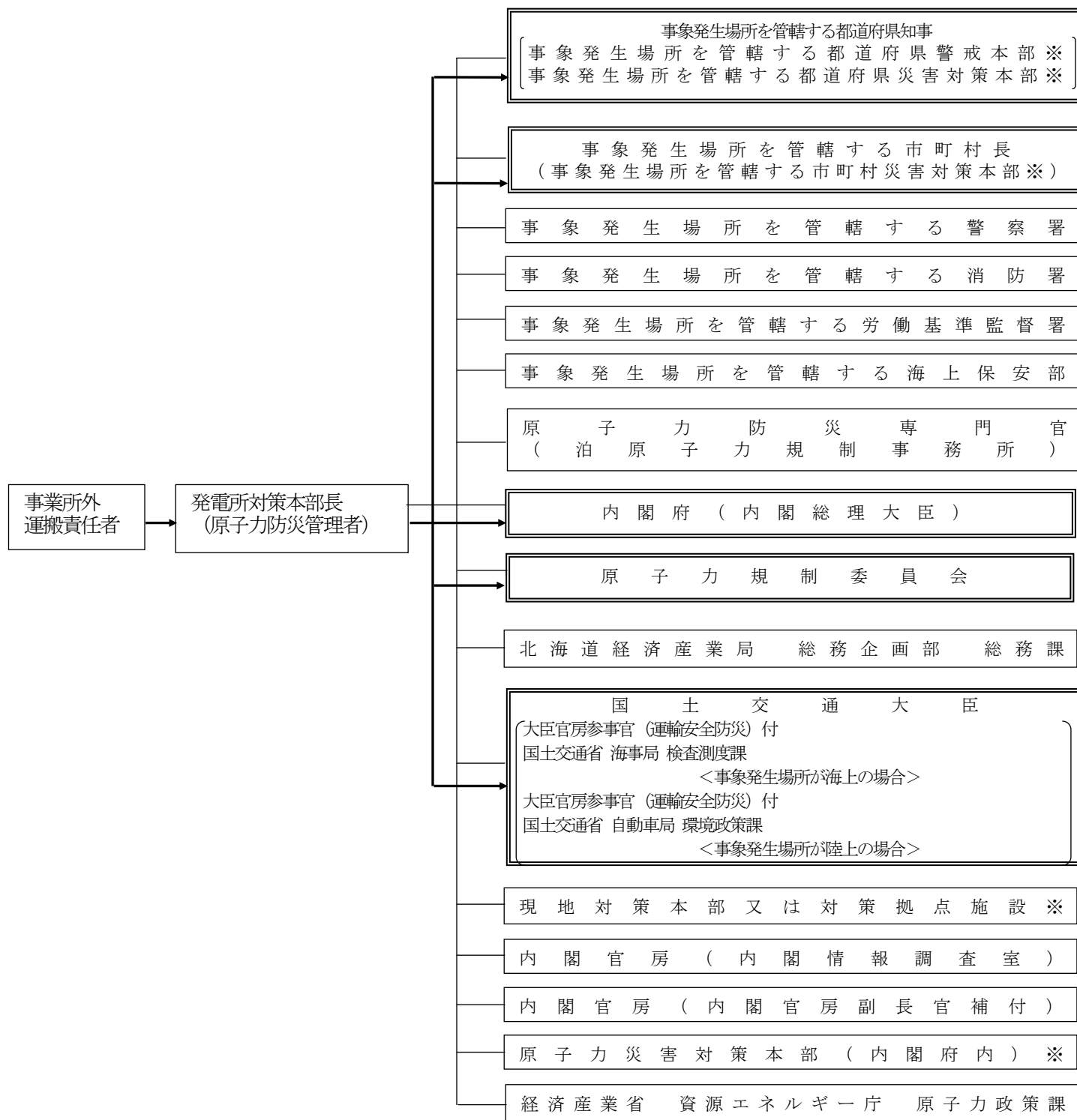
別図 3-1-3 (2) 原災法第 25 条第 2 項に基づく報告経路 (事業所外運搬での事象発生時の報告経路)
