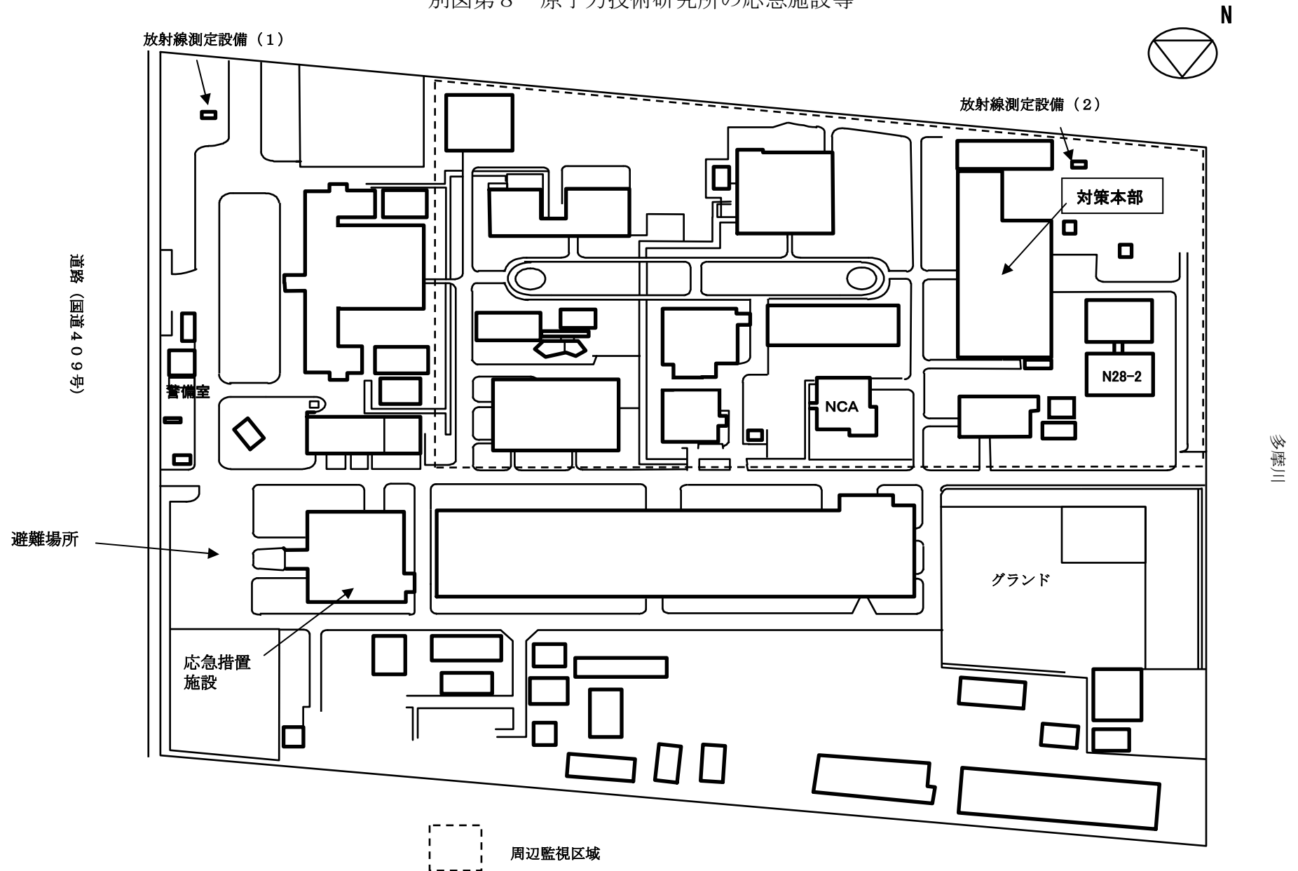
別図第8 原子力技術研究所の応急施設等
