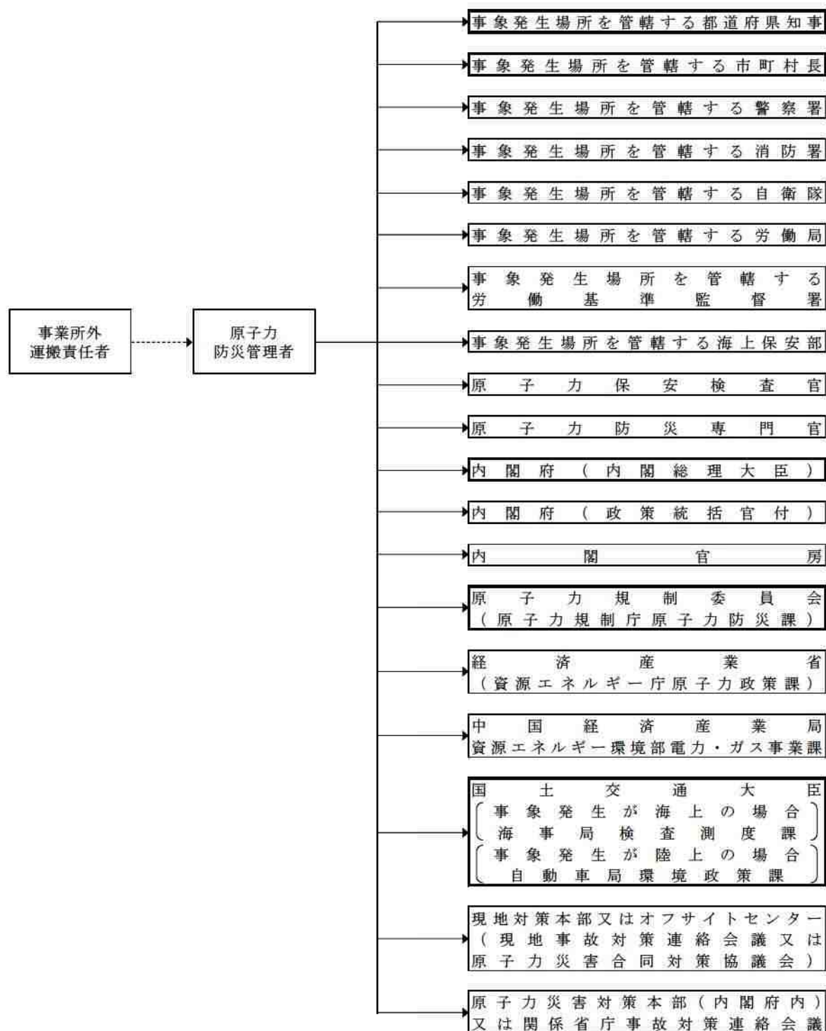
別図 5-4 原災法第10条第1項の規定に基づく通報後の連絡経路 (事業所外運搬)
