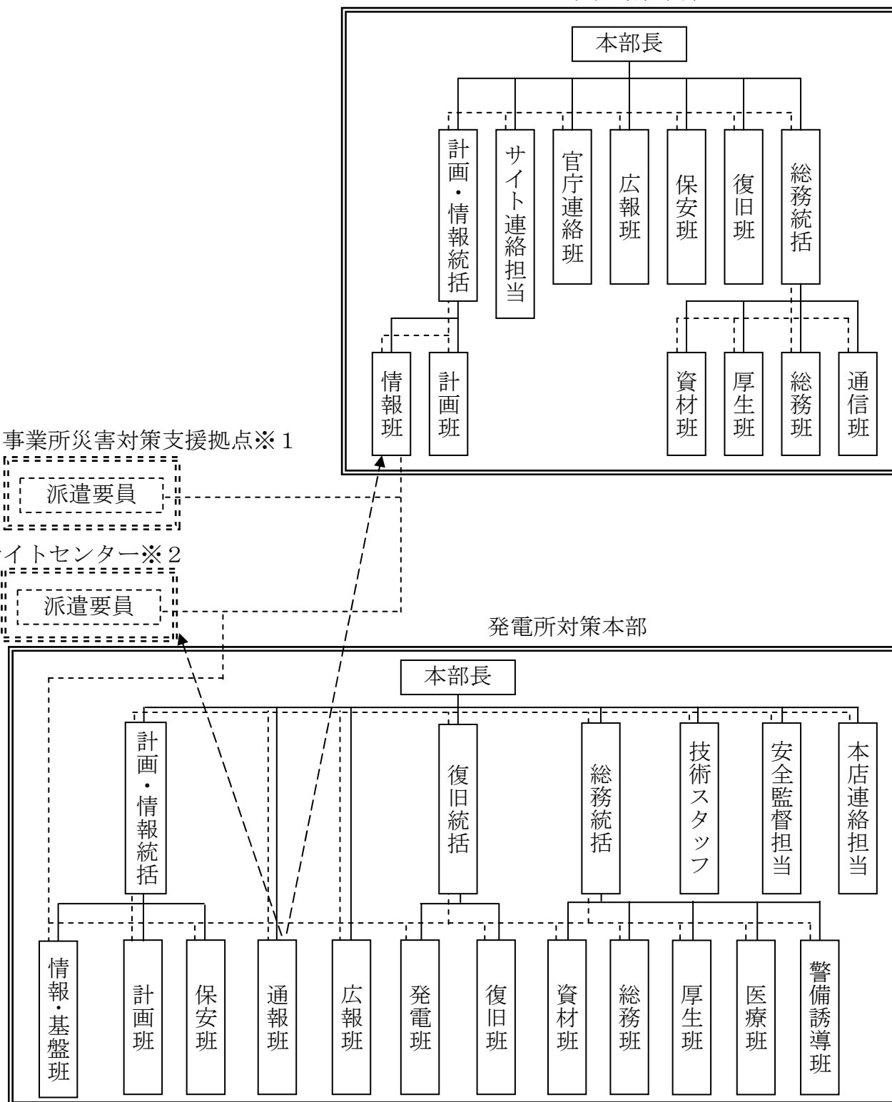
別図 2－7 緊急時態勢発令後の社内の伝達経路（第 1 次緊急時態勢発令時）（1 / 2） 本店対策本部
