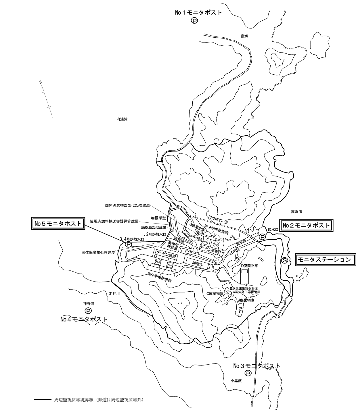
別図 2-3-1 2 発電所敷地周辺の放射線測定設備
