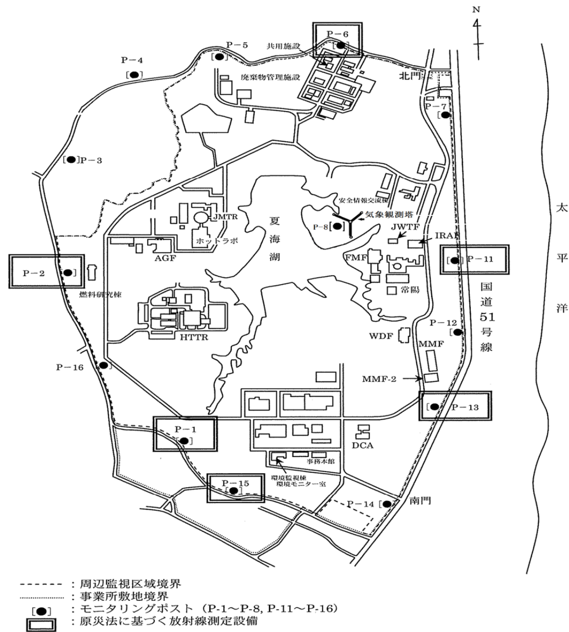
別図－4 大洗研究開発センター敷地周辺の放射線測定設備
