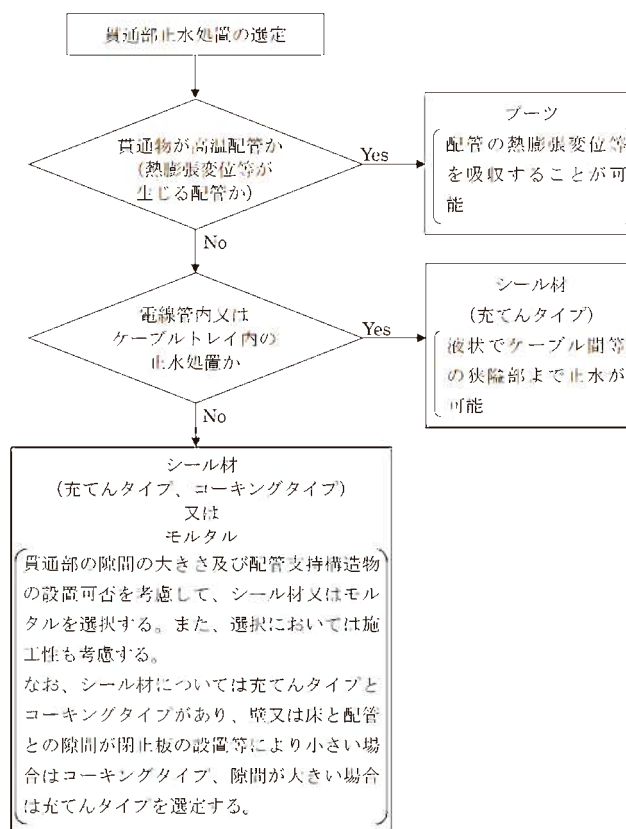
貫通部止水処置の選定フロー
