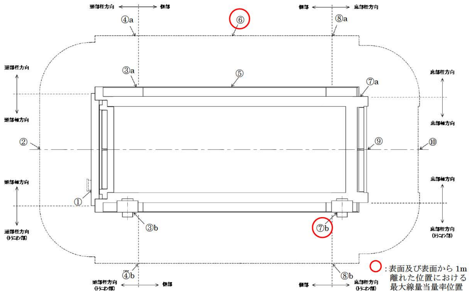
図 3-6 線量当量率評価点及び最大線量当量率位置
