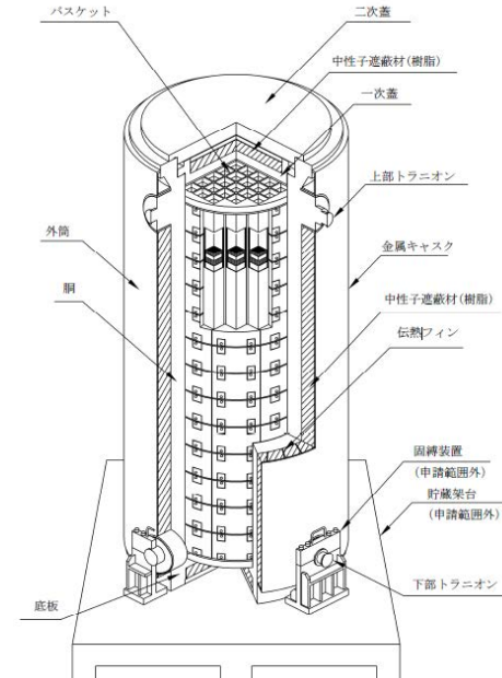
Hitz-B52型
