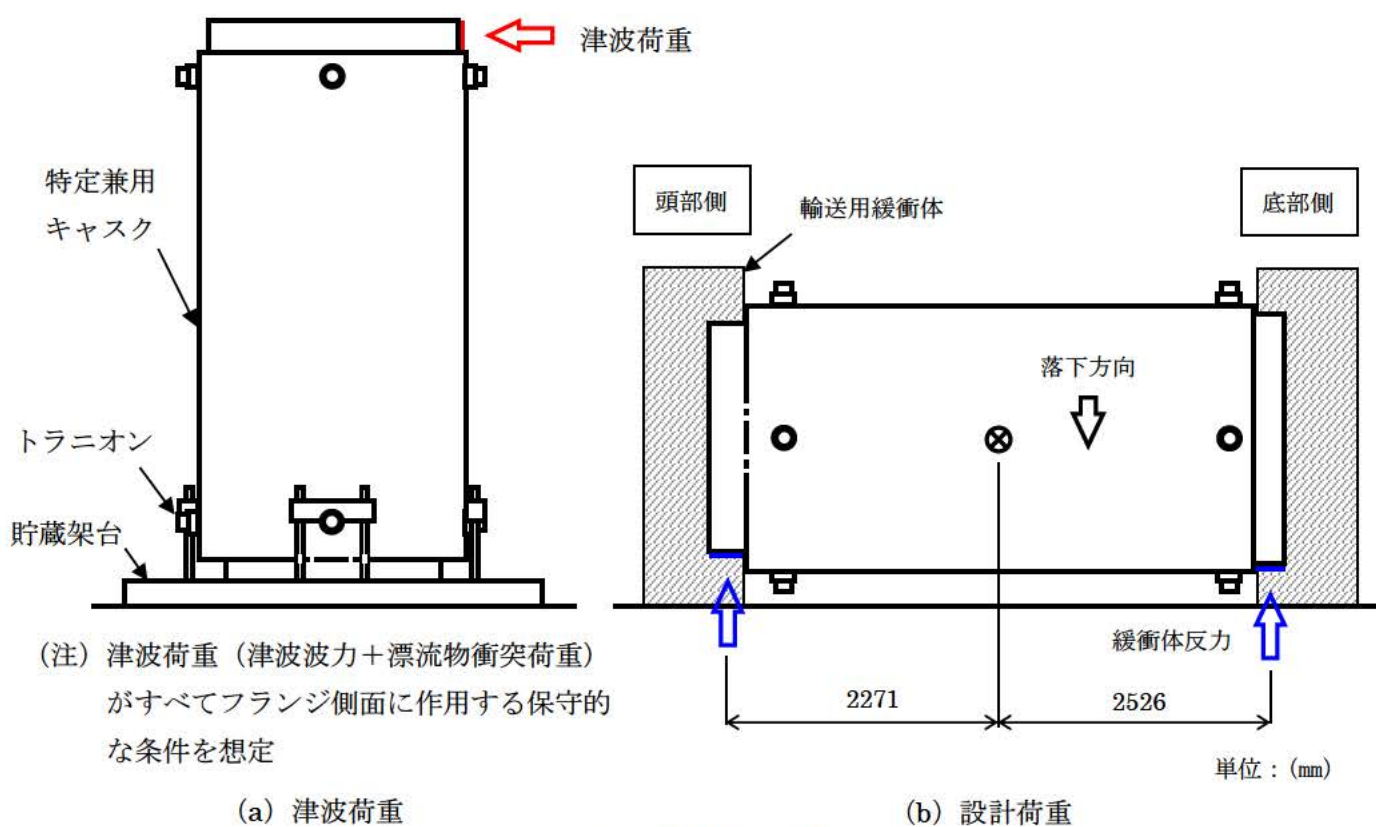
図 3 荷重作用状態の比較
