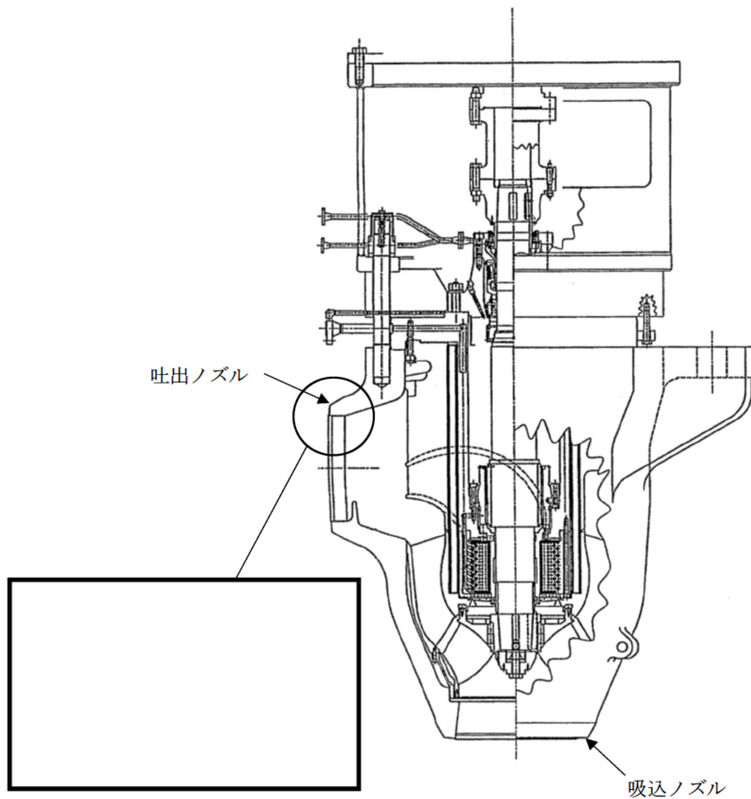
図1 1次冷却材ポンプ構造図
