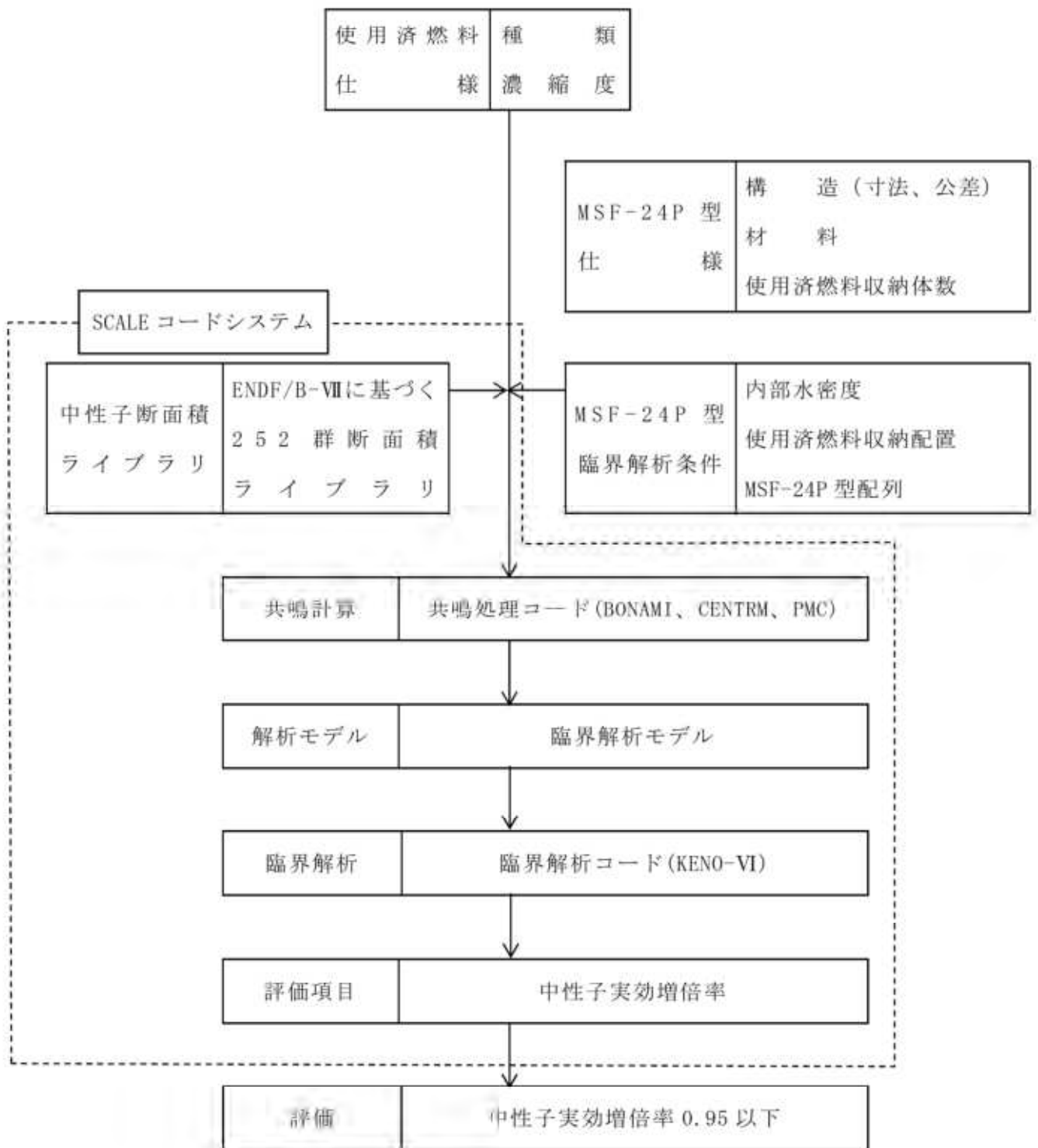
第2図 MSF-24P型の臨界解析フロー図
