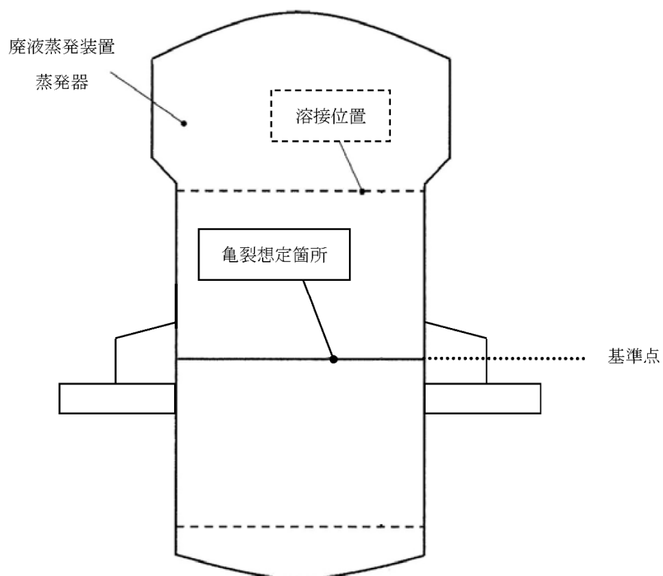
図 10-1-1 溶接位置と亀裂想定箇所
