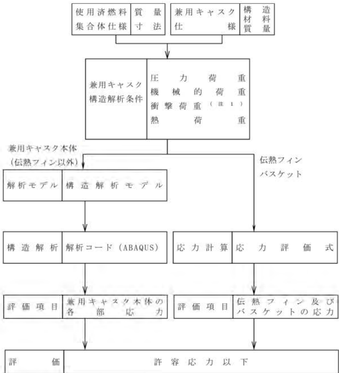
第1図 輸送時の0.3m落下時及び9m落下時の構造評価フロー (注2)
