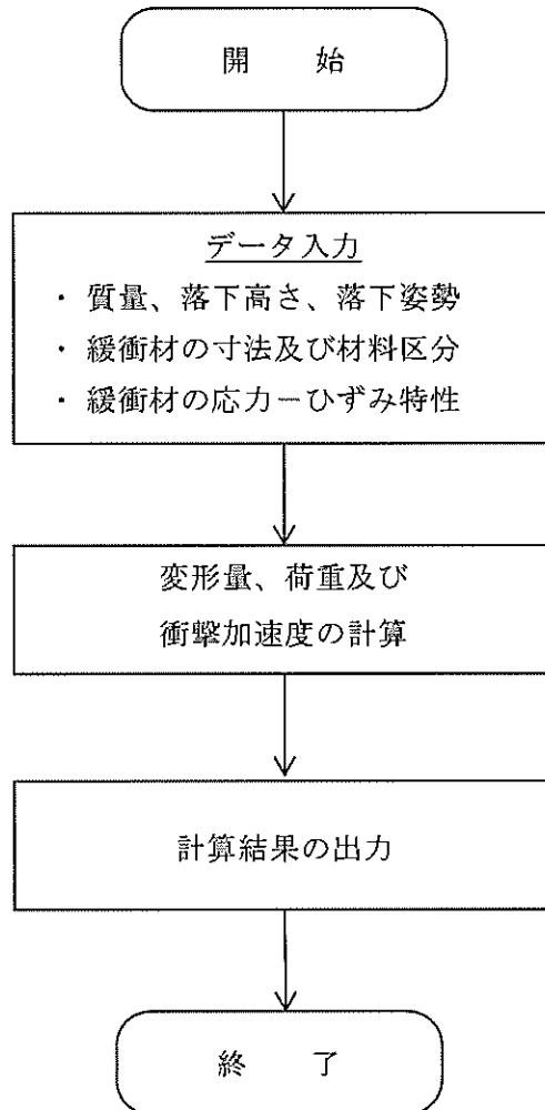
第4図 CRUSH コードの計算フロー
