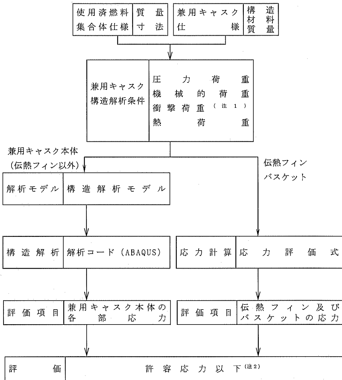
第3図 輸送時の0.3m落下時の構造評価フロー (注3)
