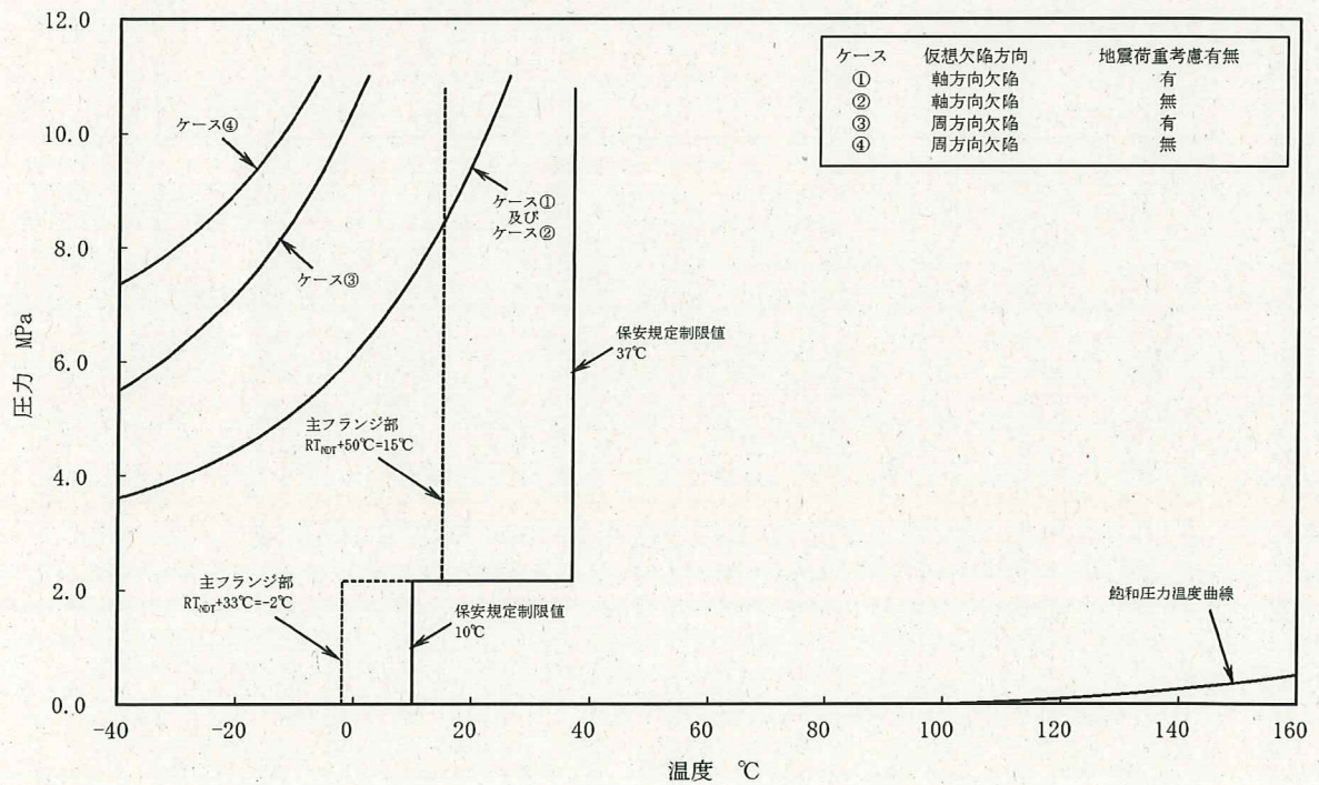
図 5-2 平成 30 年 9 月 28 日時点の原子炉压力容器の P-T 線図 (耐圧・漏えい試験時)
