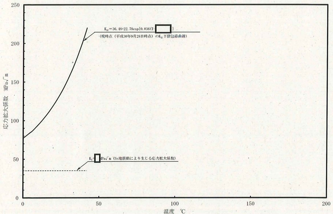
図 5-3 平成 30 年 9 月 28 日時点の K_{IC} 下限包絡曲線と K_I の関係
