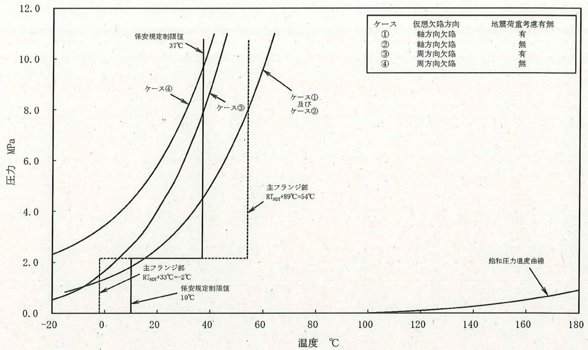
図 5-1 平成 30 年 9 月 28 日時点の原子炉压力容器の P-T 線図 (炉心臨界時)
