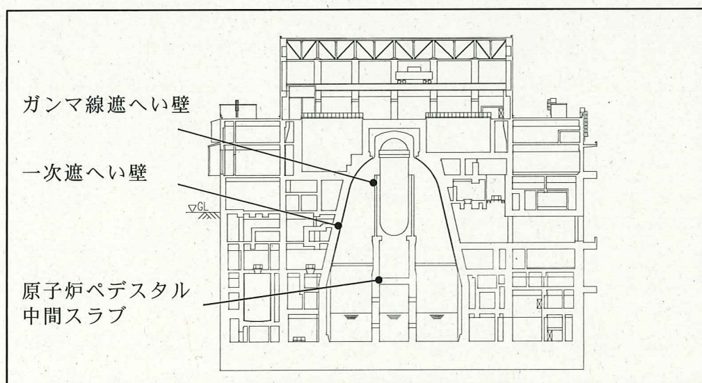
図 3 原子炉建屋の概要
