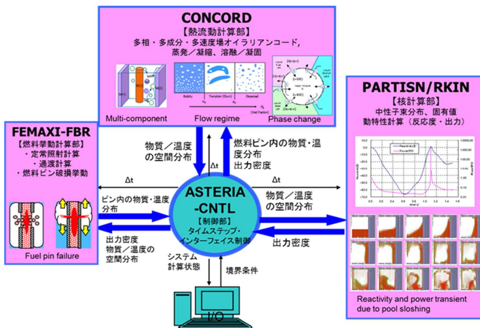
図 1 ASTERIA-FBR のコード構造
